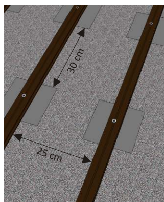
štěrkové lože
