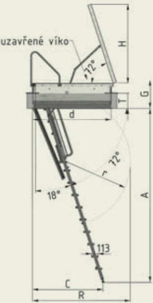
Řez dolním víkem Aristo
